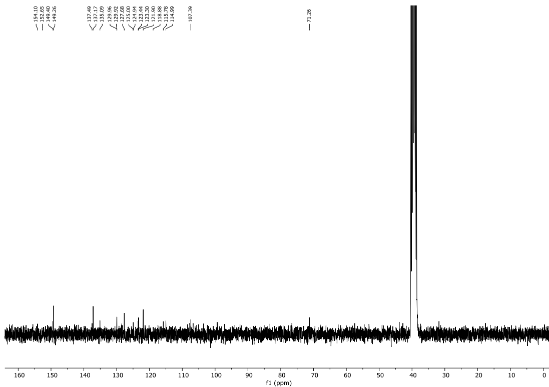
b) ^{13}\text{C} NMR spektar 2-(3-fluor-4-(piridin-2-ilmetoksi)fenil)-6-cijanobenzotiazola 9c
