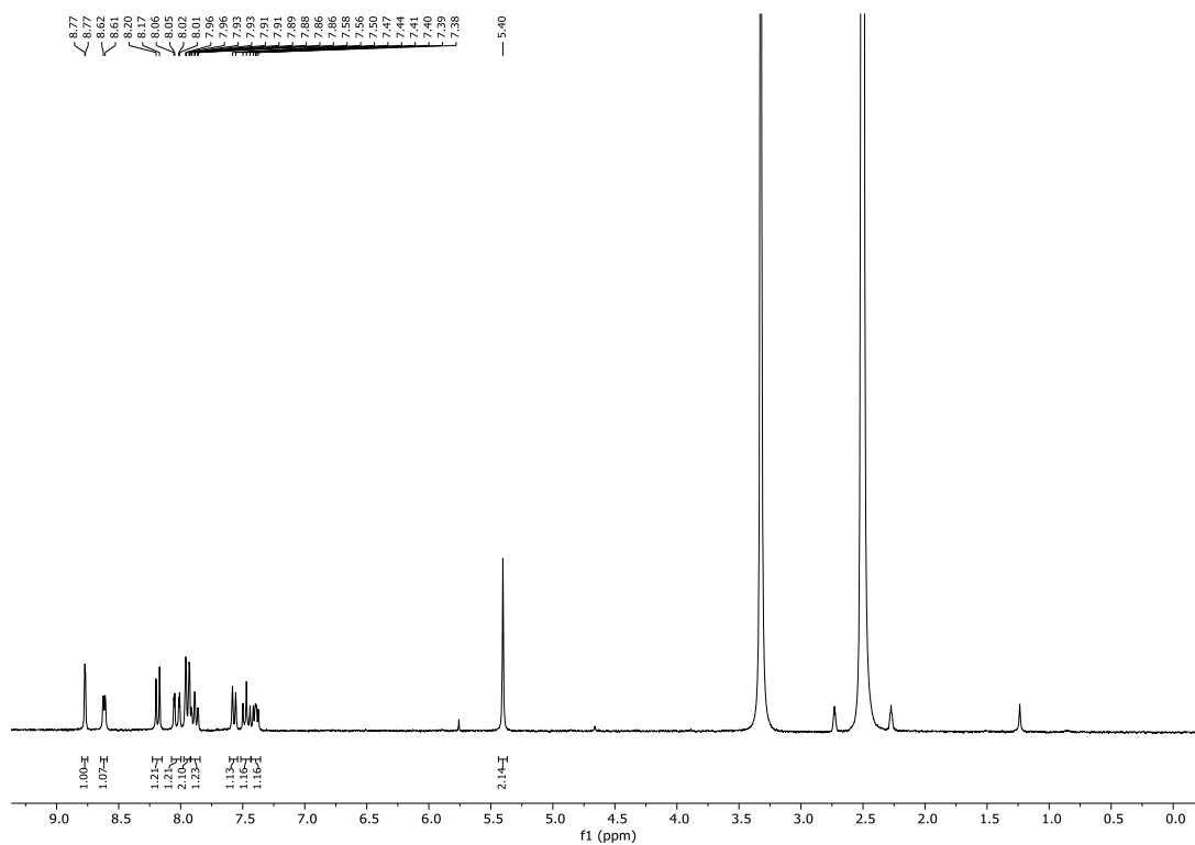
a) ^1\text{H} NMR spektar 2-(3-fluor-4-(piridin-2-ilmetoksi)fenil)-6-cijanobenzotiazola 9c
