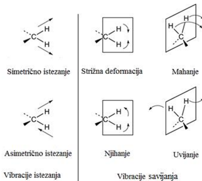
Slika 2.3.1.1. Vibracije veza istezanja i savijanja koje se mogu identificirati FTIR spektroskopijom
