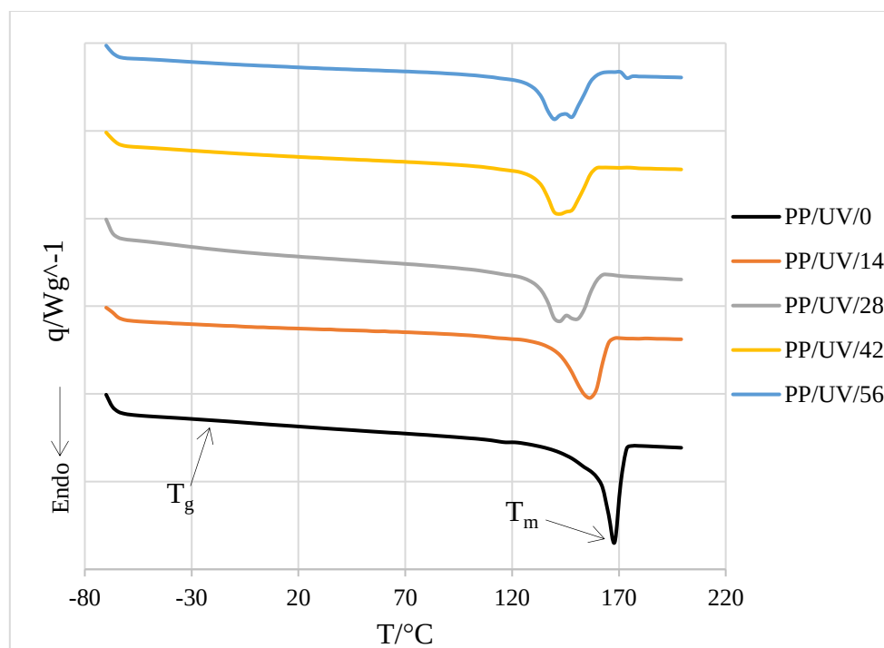
Slika 4.2.1. DSC termogrami uzoraka PP filmova UV starenih 0, 14, 28, 42 i 56 dana, temperatura taljenja ( T_m ), temperatura staklastog prijelaza ( T_g ) = -25^{\circ}\text{C}
