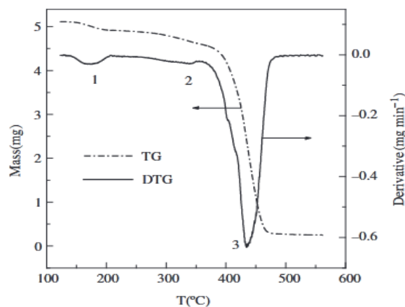
Slika 17. TG i DTG krivulja.[13]
