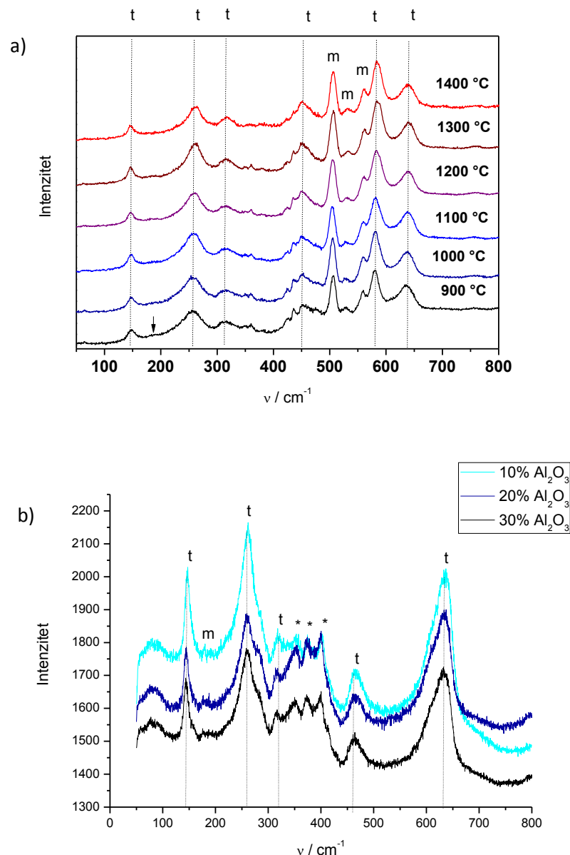
Slika 19. Ramanovi spektri: a) uzorka sgZYM kalciniranog na navedenim temperaturama i b) uzorka mkA10, mkA20 i mkA30 žarenih na 1400 °C; t – t-ZrO 2 , m – m-ZrO 2 , * – nečistoće
