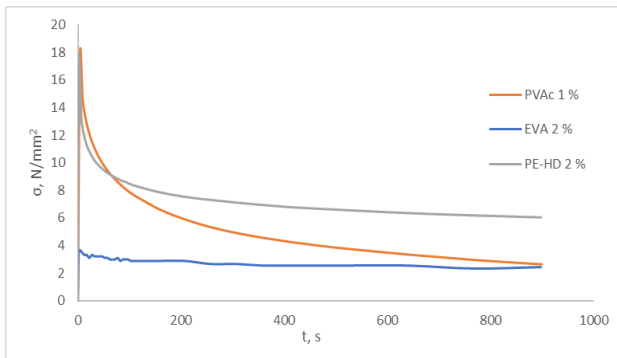
Slika 68. Ovisnost napreznja u vremenu dobivene testom relaksacije napreznja za istraživane polimere
