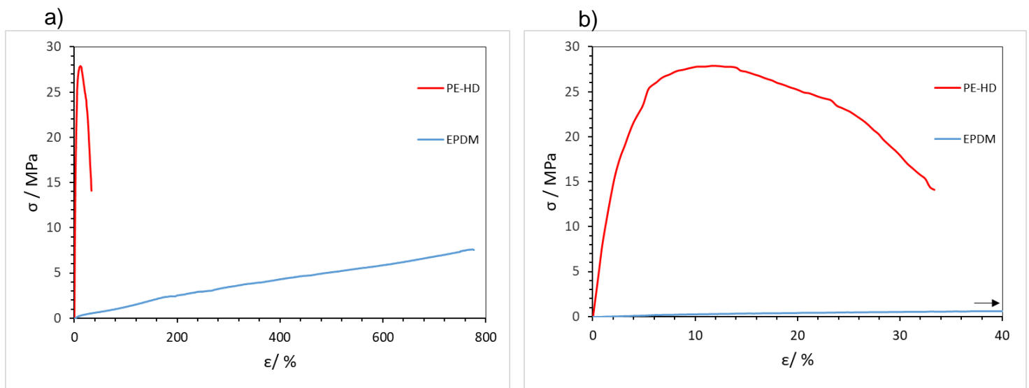
Slika 47. Krivulja naprežanje – istežanje za HD-PE i EPDM a) u cijelom području deformacija i b) u području malih deformacija
