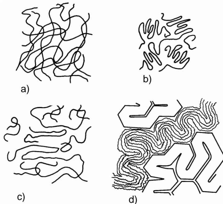
Slika 14. Nadmolekulna struktura amornih polimera; (a) model statističkog klupka, (b) konformacija statistički savijenog lanca, (c) model resastih micela od savijenih lanaca, (d) model vijugave strukture (eng. meander model)
