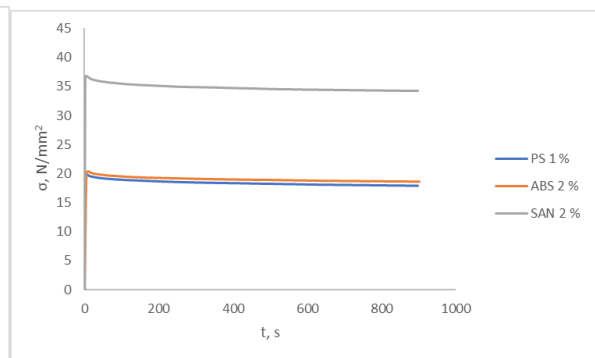
Slika 68. Ovisnost napreznja u vremenu dobivene testom relaksacije napreznja za istraživane polimere
