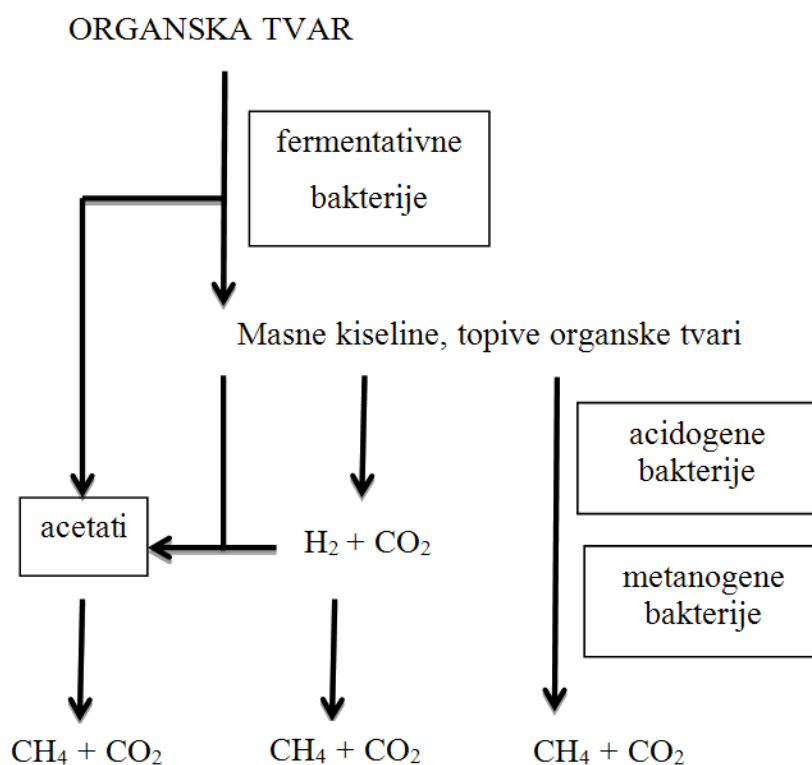
Slika 2.2. Anaerobna pretvorba organskih tvari do metana 20
