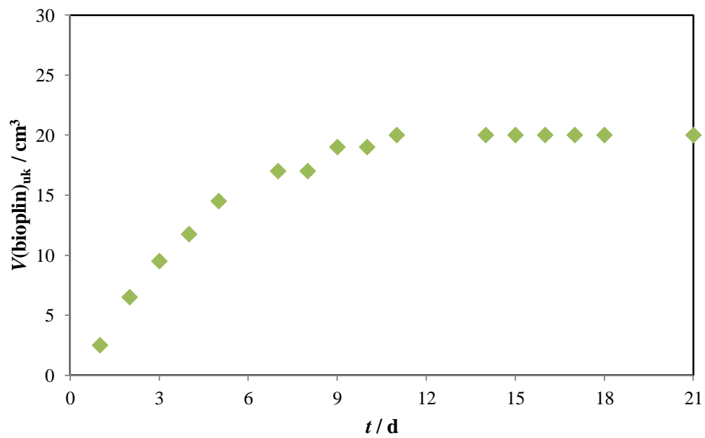
Slika 4.1. Grafički prikaz promjene kumulativnog volumena bioplina za inokulum I1 tijekom 21 dana, pri 37 °C.
