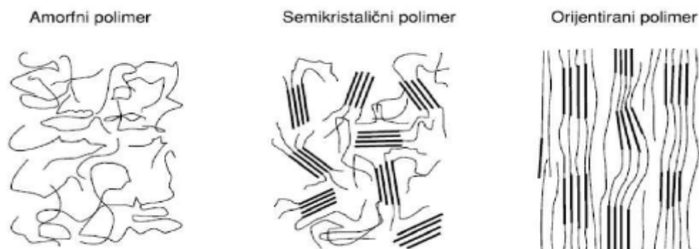
Slika 6. Podjela polimera s obzirom na nadmolekulnu strukturu.
