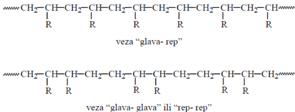
Slika 3. Modeli vezanja ponavljanih jedinica tijekom polimerizacije.
