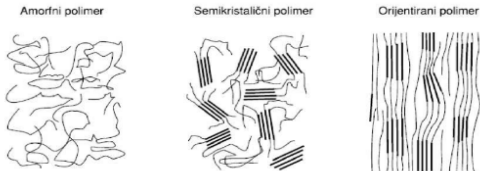
Slika 6. Podjela polimera s obzirom na nadmolekulsku strukturu.
