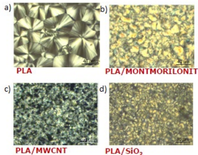
Slika 37. Smanjenje sferolita dodatkom različitih nanopunila. a) Čisti polimer. b) Dodatak montmorilonita. c) Dodatak nanocijevnica s više stijenki. d) Dodatak \text{SiO}_2 .
