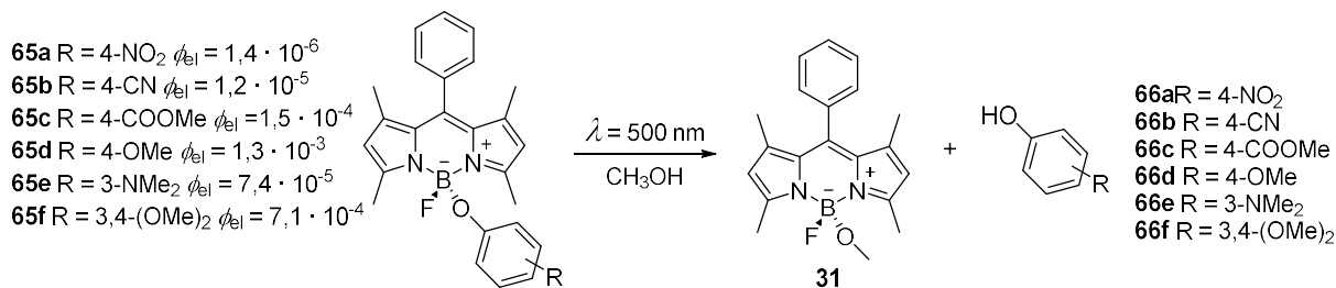
Shema 16. Fotokemijske reakcije BODIPY spojeva 65a–f s fenolnim supstituentom na borovom atomu. 68
