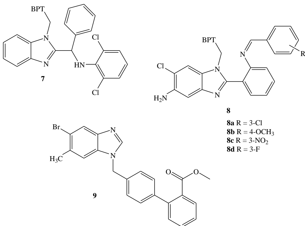
Slika 5. Derivati benzimidazola kao potencijalni antagonisti AT 1 receptora
