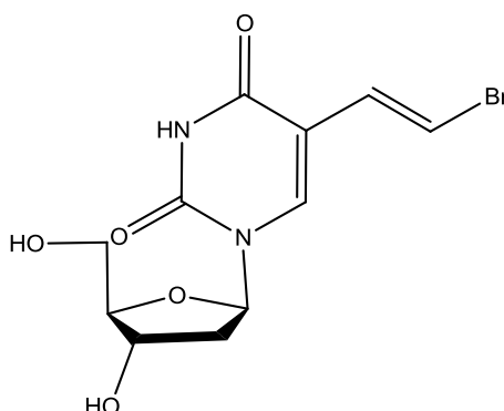
Slika 12. Struktura brivudina
