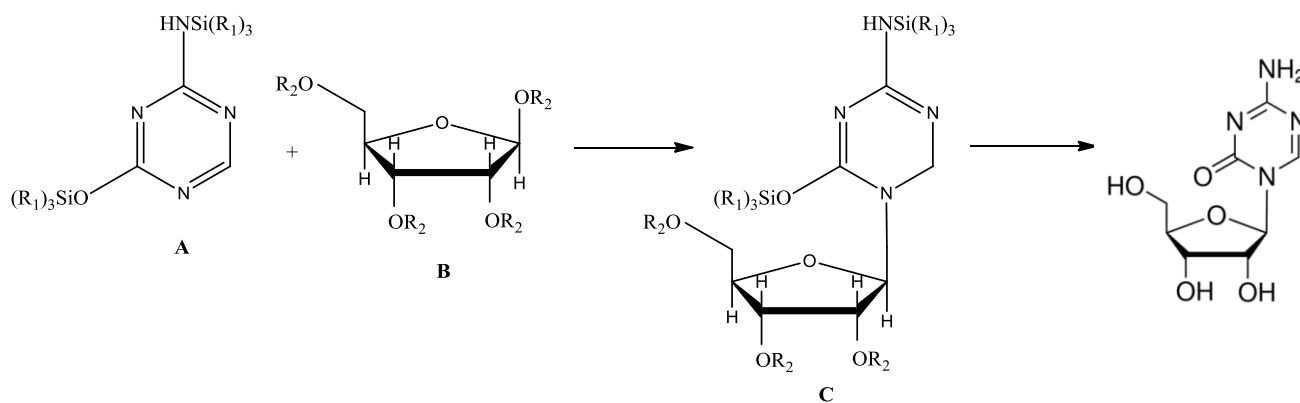
Slika 9. Sinteza 5-azacitidina
