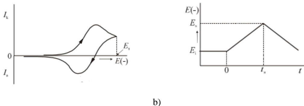
Slika 2.7 a) Voltamogram i b) Linearna ovisnost potencijala o vremenu [17]
