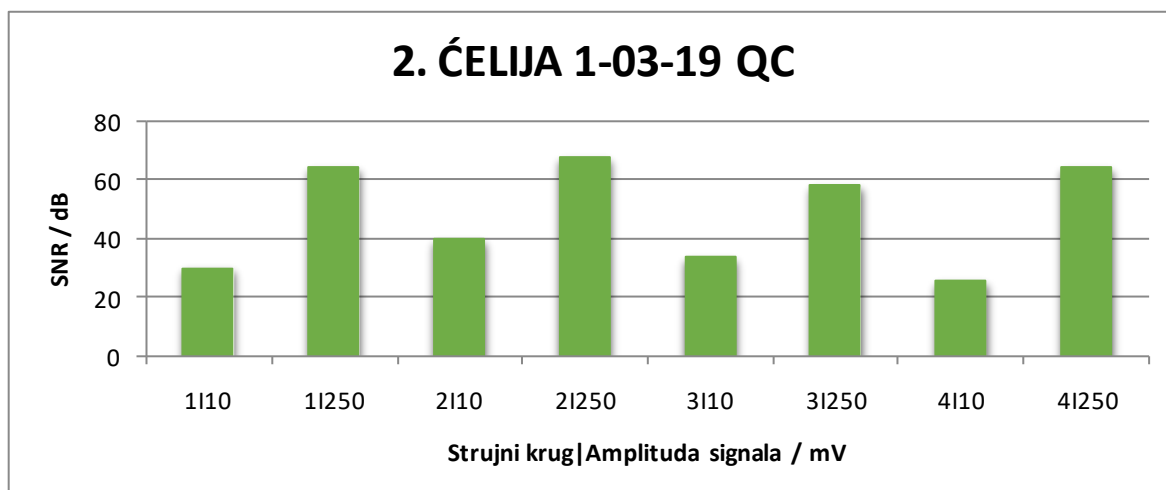
Slika 24. Omjer signala i šuma za ćeliju 1-03-19 QC u Faradayevom kavezu.
