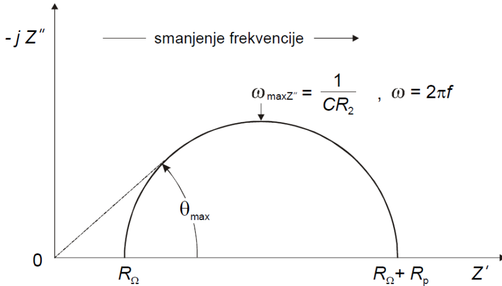
Slika 5. Nyquistov prikaz [12].
