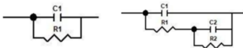
Slika 15. Ekvivalentni krugovi
