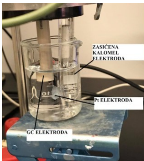
Slika 3.3. Troelektrodni sustav za redukciju sloja GO na GC elektrodi
