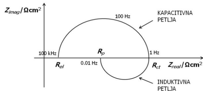
Slika 2.17. Nyquistov dijagram
