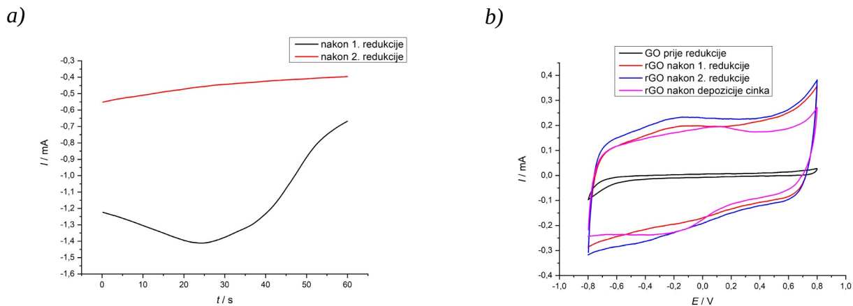
Slika 4.3. a) Kronoamperometrijski odziv zabilježen tijekom redukcije GO/10%CNT sloja na GC elektrodi u 0,1 mol \text{dm}^{-3} otopini KCl pri -1,4 V; b) ciklički voltamogrami GC/rGO10%CNT elektrode, v=50 \text{ mVs}^{-1}
