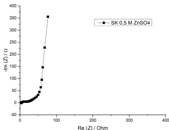
Slika 4.37. Nyquistov prikaz (rGO/20%CNT) papir/(rGO/20%CNT) papir hibridnog superkondenzatora u 0,5 mol -3 otopini ZnSO 4
