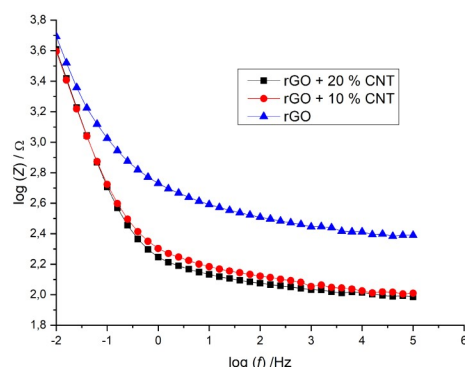
Slika 4.10. Bodeov dijagram a) ovisnosti negativnog faznog kuta o logaritmu frekvencije za GC elektrode u otopini ZnSO_4 , b) ovisnosti logaritma impedancije o logaritmu frekvencije za GC elektrode u otopini ZnSO_4
