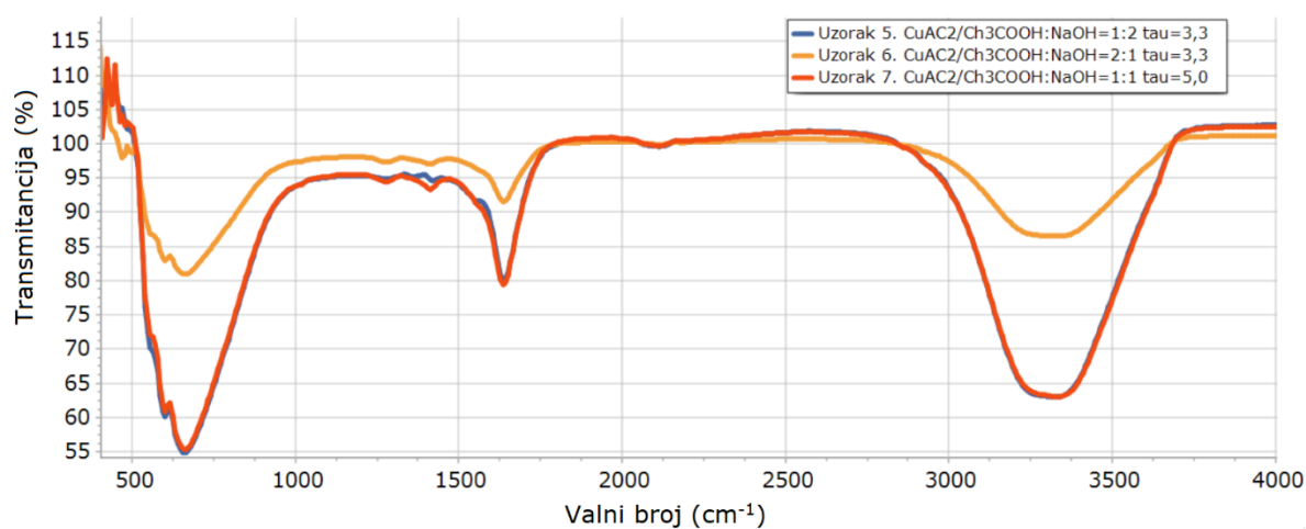
Slika 27. FTIR spektar za uzorke drugog seta sinteza
