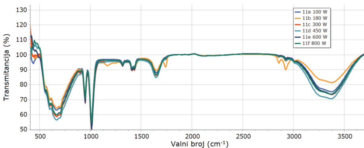
Slika 31. FTIR spektar uzorka 11 nakon pripadajućeg mikrovalnog zračenja (11A- 100 W, 11B- 180 W, 11C- 300 W, 11D- 450 W, 11E- 600 W i 11F- 800 W)
