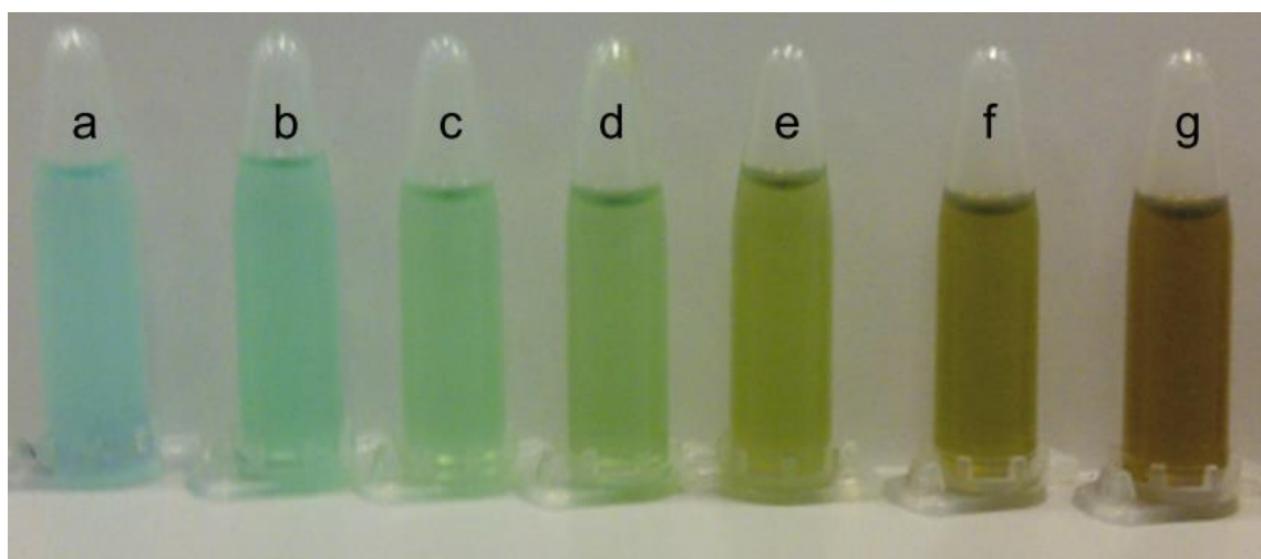
Slika 19. Postupna promjena boje otopine tijekom faza sinteze: (a) dok su se prekursori otapali, (b) 3 sata miješanja, (c) 24 sata starenja, (d - g) mikrovalnog napretka u smanjenju veličine nanočestica CuO, ponavljani su ciklusi 10, 20, 28, 34 puta
