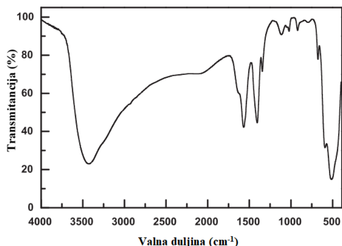
Slika 14. Prikaz FTIR spektra za CuO nanočestice [107]
