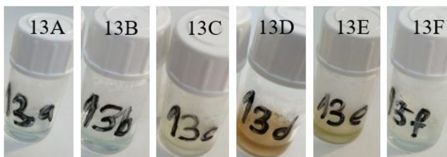
Slika 34. Uzorak 13 nakon raspodjele u 6 bočica i pripadajućeg mikrovalnog zračenja (13A- 100 W, 13B- 180 W, 13C- 300 W, 13D- 450 W, 13E- 600 W i 13F- 800 W)
