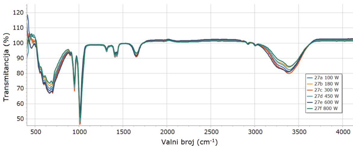
Slika 63. FTIR spektar uzorka 27 nakon pripadajućeg mikrovalnog zračenja (27A- 100 W, 27B- 180 W, 27C- 300 W, 27D- 450 W, 27E- 600 W i 27F- 800 W)
