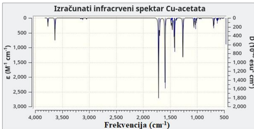
Slika 22. Izračunati FTIR spektar bakrovog (II) acetata
