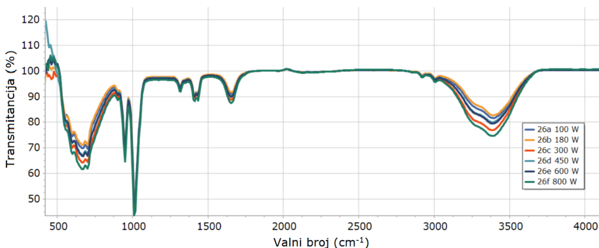
Slika 61. FTIR spektar uzorka 26 nakon pripadajućeg mikrovalnog zračenja (26A- 100 W, 26B- 180 W, 26C- 300 W, 26D- 450 W, 26E- 600 W i 26F- 800 W)
