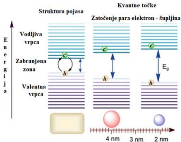
Slika 5. Prikaz efekta kvantnog ograničavanja, pri čemu se razmak između valentne i vodljive vrpce povećava, dok se veličina materijala smanjuje na kvantnu razinu zbog zadržavanja elektronske šupljine koje ostaju ograničene u diskretnoj valentnoj vrpci, a elektroni u diskretnoj vodljivoj vrpci. [54]
