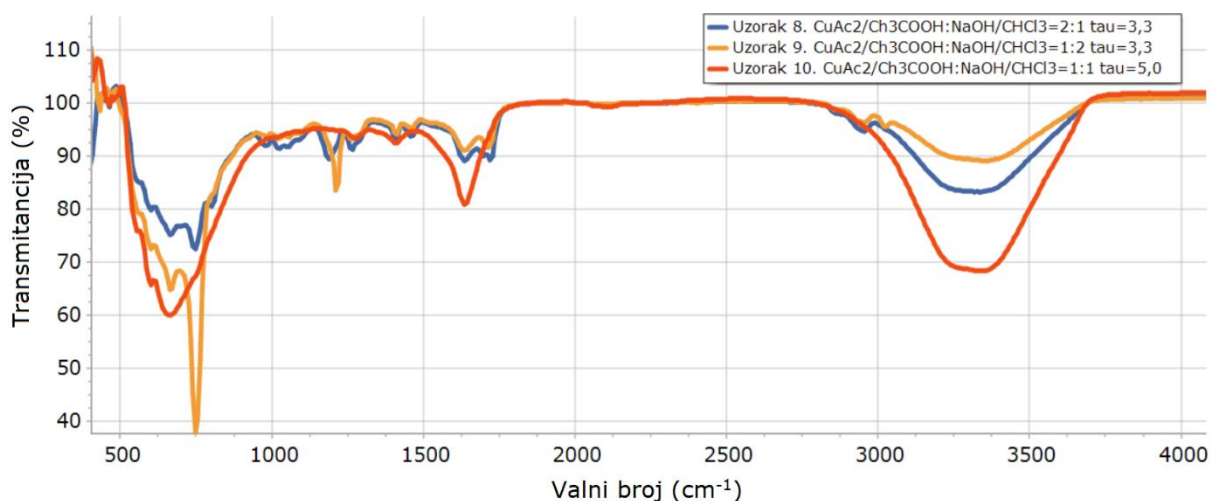
Slika 28. Uzorci iz trećeg seta sinteza
