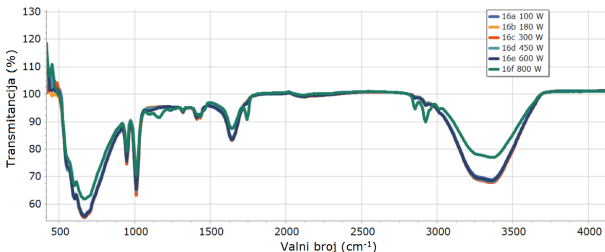
Slika 40. Uzorak 16 nakon raspodjele u 6 bočica i pripadajućeg mikrovalnog zračenja (16A- 100 W, 16B- 180 W, 16C- 300 W, 16D- 450 W, 16E- 600 W i 16F- 800 W)
