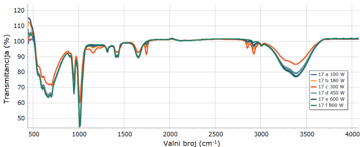
Slika 42. Uzorak 17 nakon raspodjele u 6 bočica i pripadajućeg mikrovalnog zračenja (17A- 100 W, 17B- 180 W, 17C- 300 W, 17D- 450 W, 17E- 600 W i 17F- 800 W)
