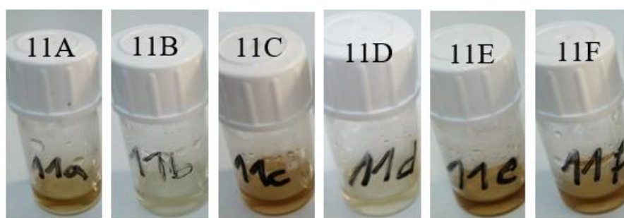
Slika 30. Uzorak 11 nakon raspodjele u 6 bočica i pripadajućeg mikrovalnog zračenja (11A- 100 W, 11B- 180 W, 11C- 300 W, 11D- 450 W, 11E- 600 W i 11F- 800 W)
