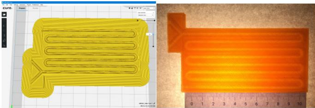
Slika 15. Prikaz lijevo: poprečni presjek iz programa za „slikanje“ Cura 4.0; Prikaz desno: izrađeni milireaktori s dva oblika ulazne sekcije.
