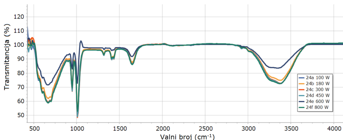
Slika 56. Uzorak 24 nakon raspodjele u 6 bočica i pripadajućeg mikrovalnog zračenja (24A- 100 W, 24B- 180 W, 24C- 300 W, 24D- 450 W, 24E- 600 W i 24F- 800 W)
