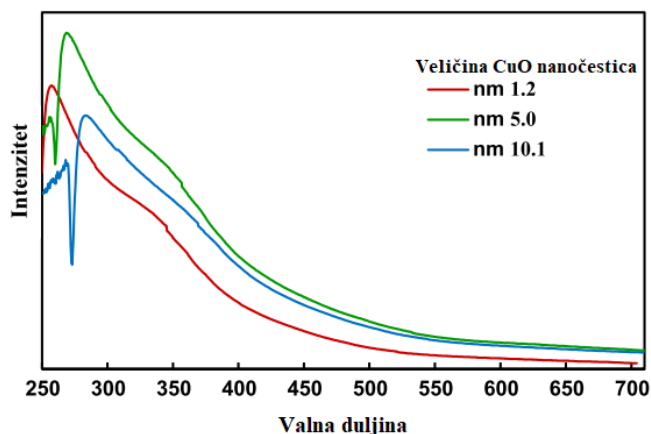
Slika 12. UV/VIS spektar CuO nanočestica [90]
