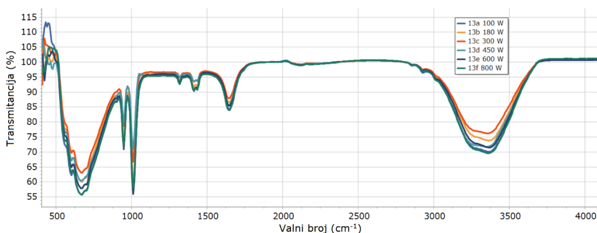
Slika 35. FTIR spektar uzorka 13 nakon pripadajućeg mikrovalnog zračenja (13A- 100 W, 13B- 180 W, 13C- 300 W, 13D- 450 W, 13E- 600 W i 13F- 800 W)
