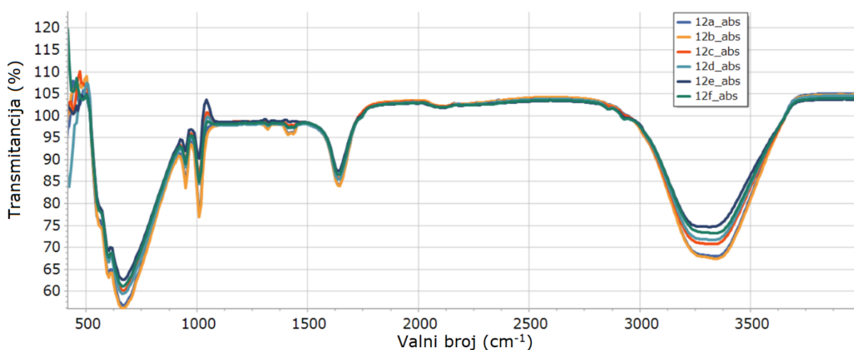
Slika 33. FTIR spektar uzorka 12 nakon pripadajućeg mikrovalnog zračenja (12A- 100 W, 12B- 180 W, 12C- 300 W, 12D- 450 W, 12E- 600 W i 12F- 800 W)
