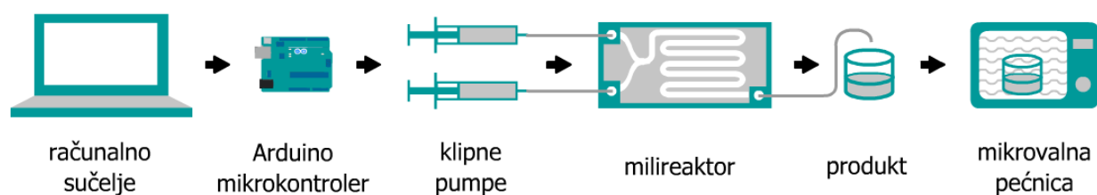
Slika 16. Shematski prikaz procesa sinteze pomoću milireaktora potpomognute mikrovalnim zračenjem.
