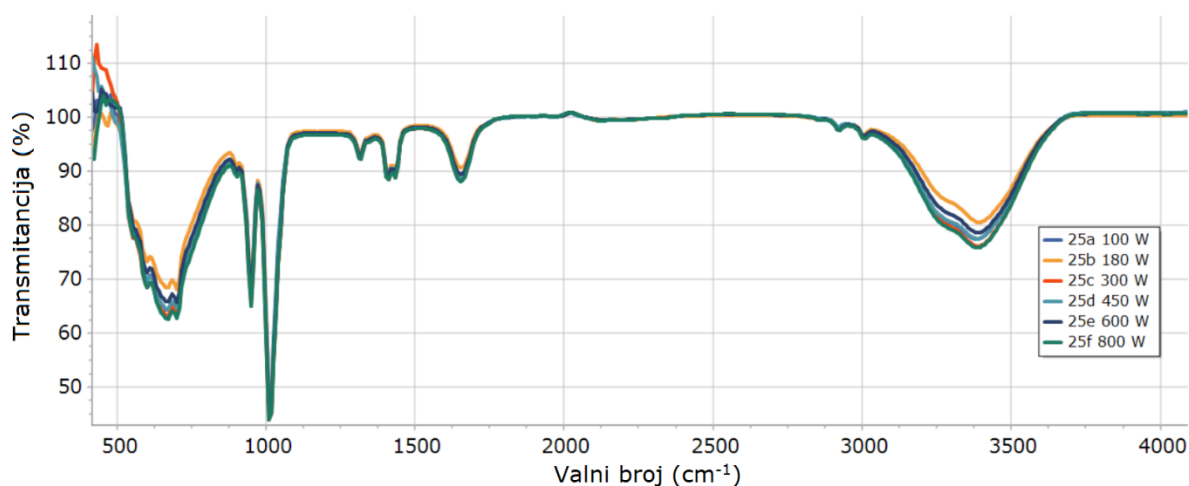
Slika 59. FTIR spektar uzorka 25 nakon pripadajućeg mikrovalnog zračenja (25A- 100 W, 25B- 180 W, 25C- 300 W, 25D- 450 W, 25E- 600 W i 25F- 800 W)
