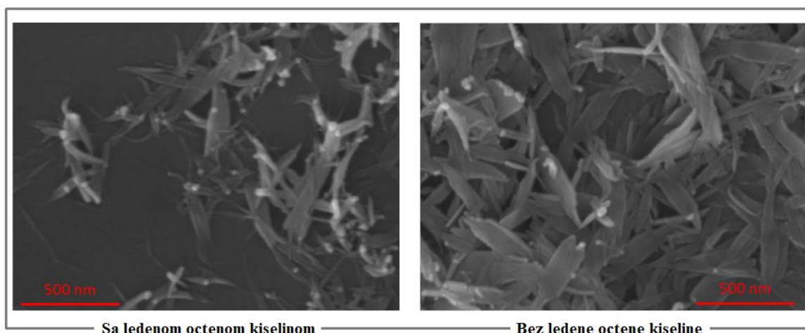
Slika 25. Prikaz SEM rezultata za uzorke sa i bez ledene octene kiseline [115]
