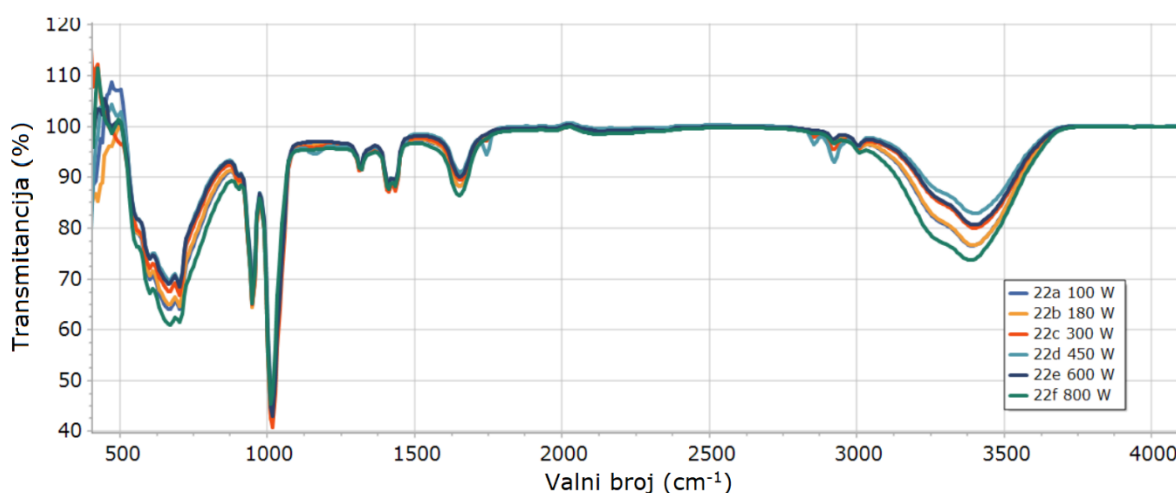
Slika 52. Uzorak 22 nakon raspodjele u 6 bočica i pripadajućeg mikrovalnog zračenja (22A- 100 W, 22B- 180 W, 22C- 300 W, 22D- 450 W, 22E- 600 W i 22F- 800 W)
