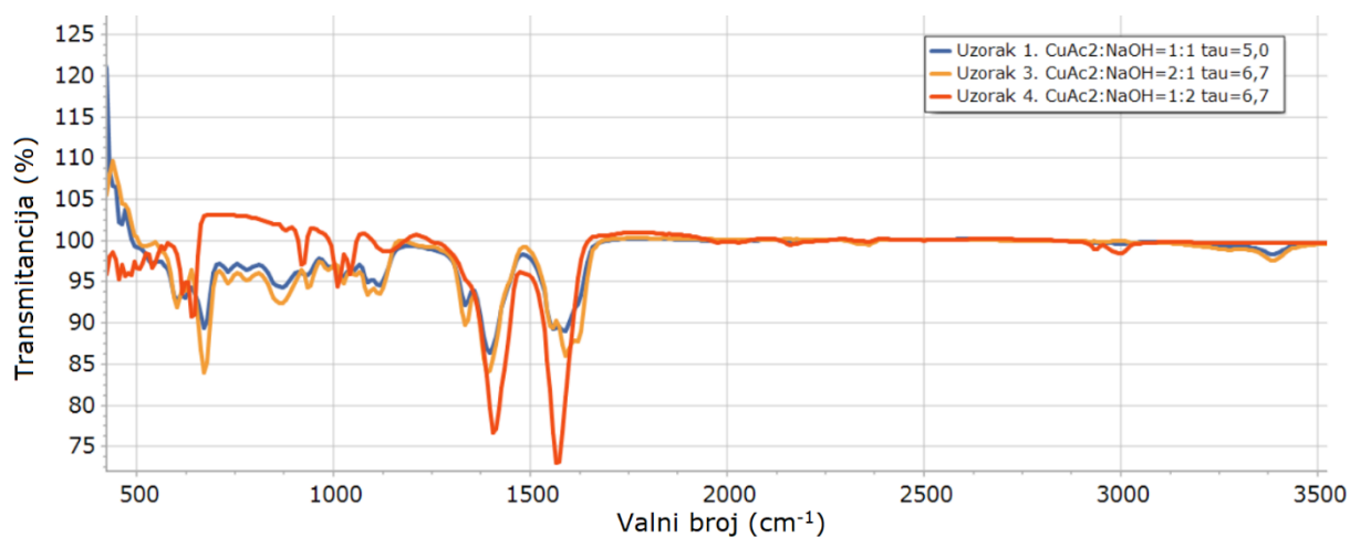
Slika 23. Uzorci prvog seta sinteza nakon mikrovalnog zračenja
