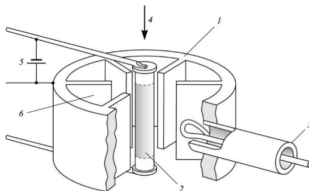
Slika 7. Dijelovi magetrona: 1. anoda, 2. katoda, 3. koaksijalna linija na izlazu, 4. smjer magnetskoga polja, 5. anodni napon, 6. rezonantna šupljina [87]
