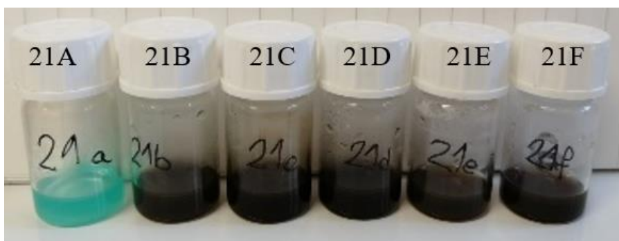
Slika 50. Uzorak 21 nakon raspodjele u 6 bočica i pripadajućeg mikrovalnog zračenja (21A- 100 W, 21B- 180 W, 21C- 300 W, 21D- 450 W, 21E- 600 W i 21F- 800 W)
