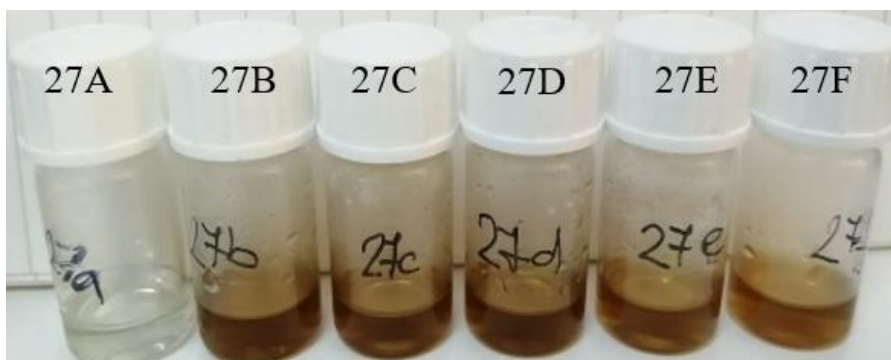
Slika 62. Uzorak 27 nakon raspodjele u 6 bočica i pripadajućeg mikrovalnog zračenja (27A- 100 W, 27B- 180 W, 27C- 300 W, 27D- 450 W, 27E- 600 W i 27F- 800 W)
