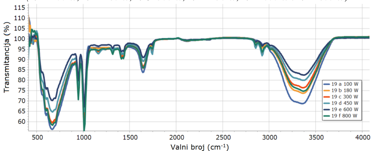
Slika 46. Uzorak 19 nakon raspodjele u 6 bočica i pripadajućeg mikrovalnog zračenja (19A- 100 W, 19B- 180 W, 19C- 300 W, 19D- 450 W, 19E- 600 W i 19F- 800 W)
