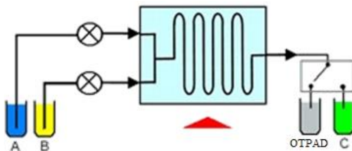
Slika 9. Shema milireaktora sa dva ulaza i jednim izlazom. [100]
