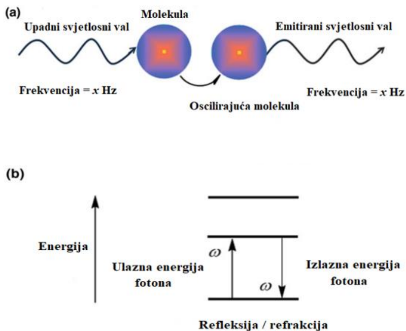
Slika 3. Prikaz linearnog optičkog sustava: a) nema promjene u frekvenciji upadnog svjetlosnog vala nakon emitiranja vibracijom molekule s kojom je djelovala i b) bez promjene energije fotona nakon istog događaja [54]
