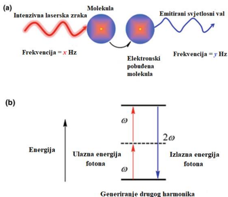
Slika 4. Prikaz nelinearnog optičkog sustava; a) promjena frekvencije ulaznog svjetlosnog vala nakon što ga emitira vibracijska molekula s kojom je stupila u interakciju i b) promjena energije fotona nakon istog događaja, primjer generiranja drugog harmonika. [54]
