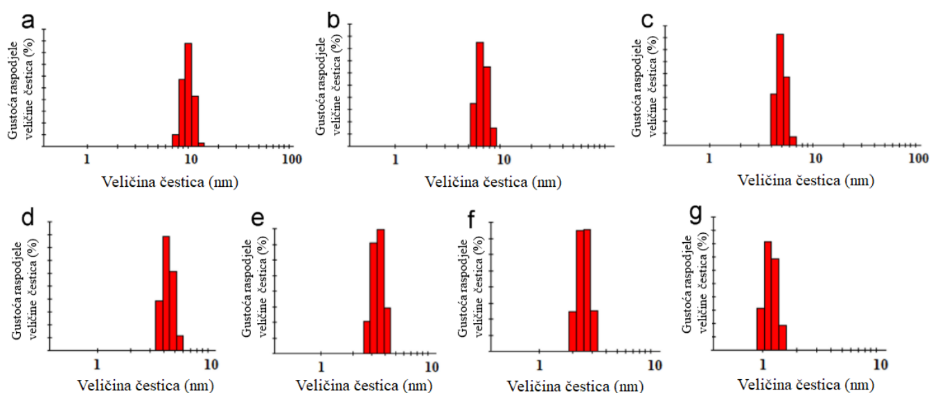
Slika 20. Histogrami raspodjele veličine koloidnih nanočestica CuO, radni ciklus mikrovalne pećnice ponavljen je (a) 20, (b) 24, (c) 28, (d) 30, (e) 32, (f) 34 i (g) 36 puta.
