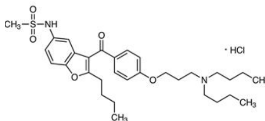
Slika 10. Struktura dronedaron-hidroklorida
