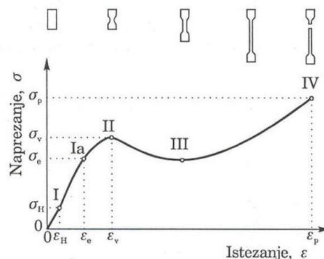
Slika 18. Karakteristična područja naprežanje istežanje.
