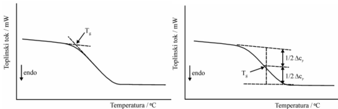
Slika 15. Primjer određivanja staklišta iz DSC krivulje
