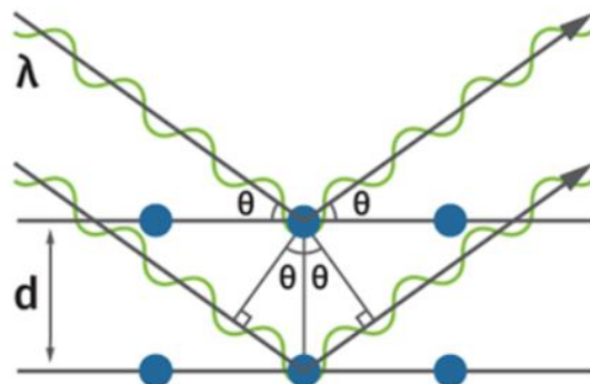
Slika 5. Princip difrakcije rendgenskih zraka na kristalu. 18,19
