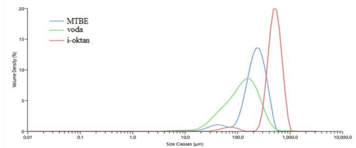
Slika 4.9. Utjecaj antiotapala na raspodjelu veličina i oblik kristala pri naglom dodatku antiotapala
