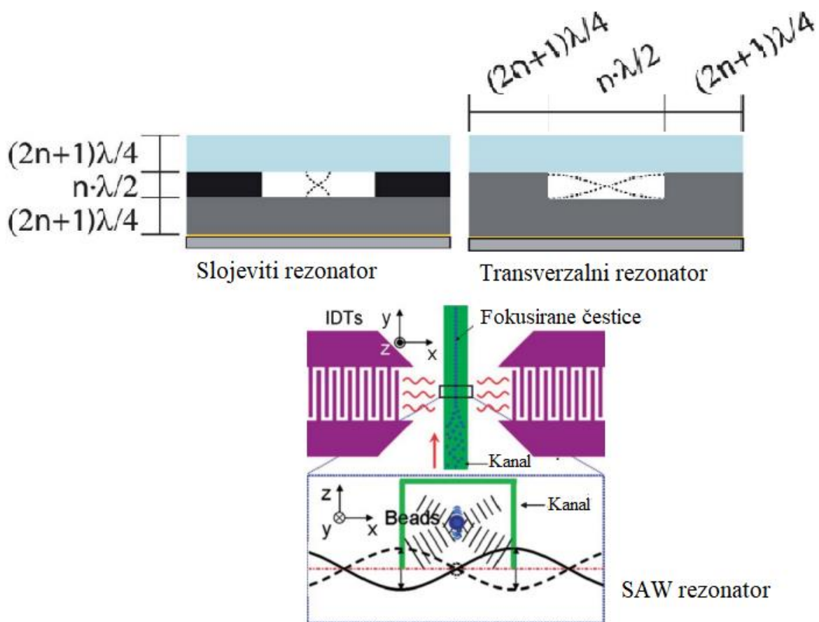
Slika 40. Usporedba slojevitog, transverzalnog i SAW rezonatora
