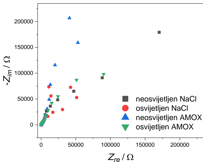
Slika 4.16 Grafički prikaz impedancijskih odziva (Nyquistov dijagram) za \text{TiO}_2/\text{SnS}_2 elektrodu pri potencijalu E=0,5 V za otopinu 0,1 \text{ mol dm}^{-3} NaCl i otopinu 0,1 \text{ mmol dm}^{-3} farmaceutika Amoxicilin u 0,1 \text{ mol dm}^{-3} NaCl.
