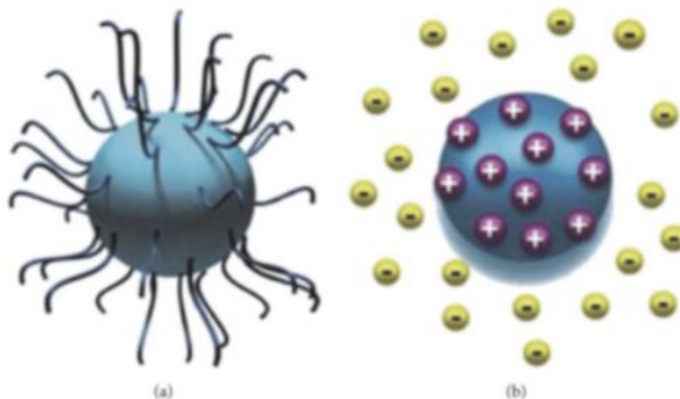
Slika 9. Mehhanizmi odbijanja: (a) sterička odbojnost i (b) elektrostatička odbojnost [23]
