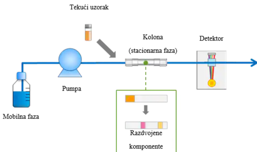
Slika 3.7. Shematski prikaz kapljene kromatografije visoke djelotvornosti. 15
