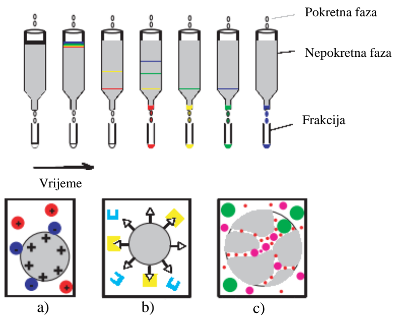
Slika 4. Princip kromatografije: a) ionska b) afinitetna c) gel
