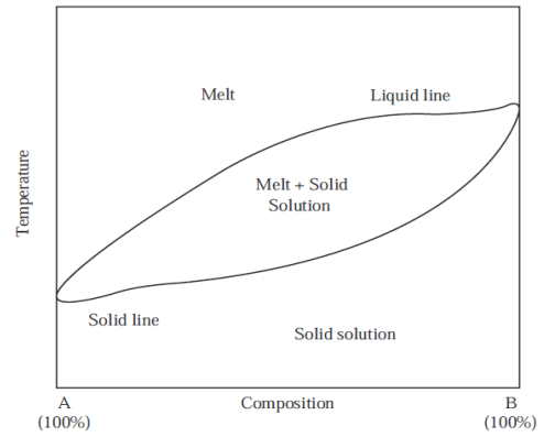
Slika 2. Fazni dijagram kontinuirane čvrste otopine 9
