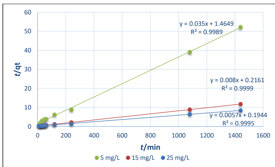
Slika 14. Grafički prikaz pseudokinetičkog modela II. reda
