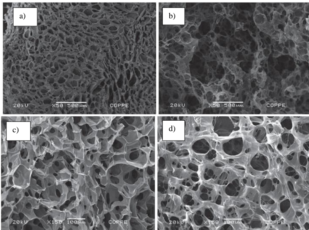
Slika 4.3. SEM mikrografi a) i c) kitozana, b) i d) kitozan modificiran kolagenom pri različitom povećanju
