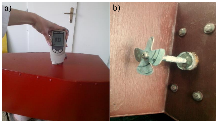
Slika 21. a) mjerenje debljine premaza, b) instalirana osovina i propeler
