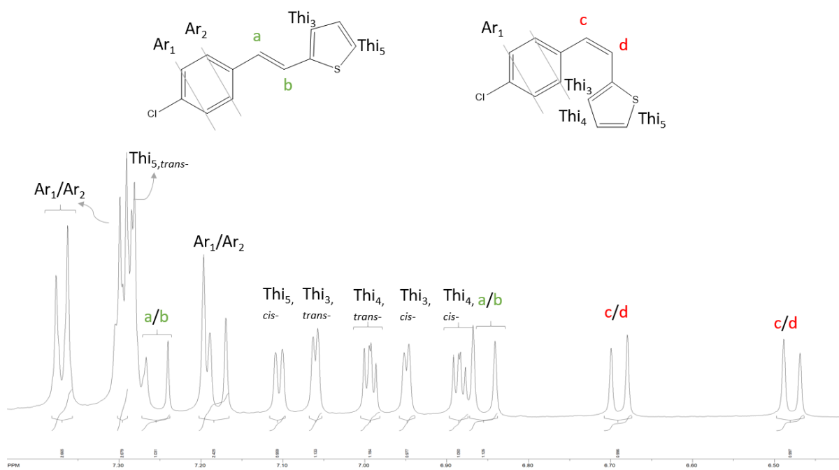
Slika 7. Uvećani prikaz ^1\text{H} NMR spektra 2-(4-klorostiril)tiofena ( I ).
