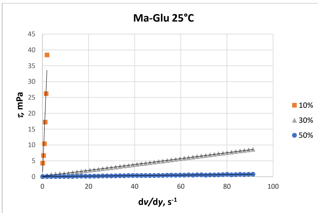
Slika 13. Promjena smičnog naprezanja Ma-Glu s različitim masenim udjelima vode u ovisnosti o promjeni smične brzine pri temperaturi od 25 °C.
