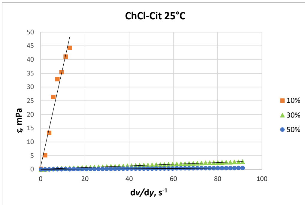
Slika 12. Promjena smičnog naprezanja ChCl-Cit s različitim masenim udjelima vode u ovisnosti o promjeni smične brzine pri 25 °C.
