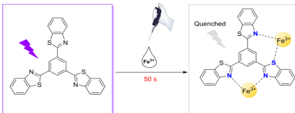
Slika 26. Shema reakcijskog mehanizma 40
