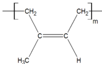
Slika 5. Primjer cis-polimera 2
