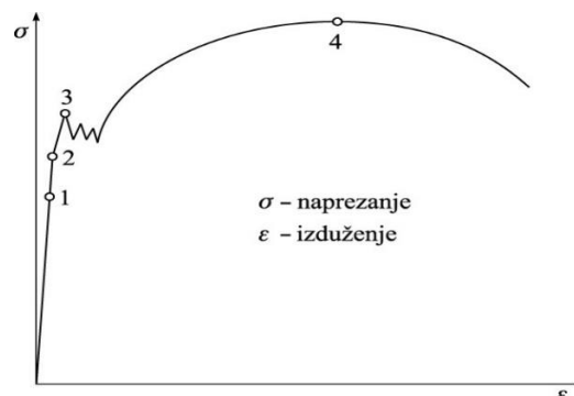
Slika 25. Dijagram naprezanje-deformacija [9]
