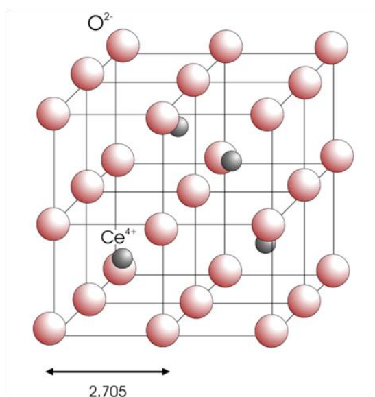
Slika 1. Shematski prikaz jedinične ćelije CeO 2 [5]
