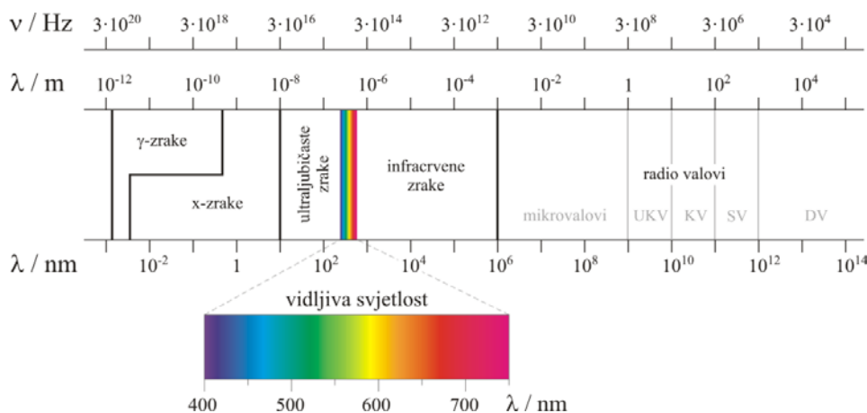
Slika 4.9. Prikaz spektra elektromagnetskog zračenja
