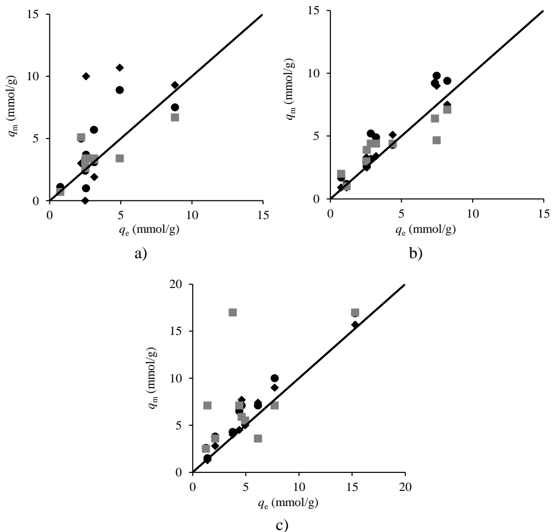
Slika 45 Odnos adsorpcijskih parametara q_m iz Langmuirve (●), Dubinjin-Raduškjevičeve (◆) i Hillove izoterme (■) naspram eksperimentalno određenih adsorpcijskih kapaciteta polifenola q_e . Prikazani rezultati odnose se za početne koncentracije od 150 mg/L, pri : a) pH 1,5; b) pH 5,5; c) pH 10,0
