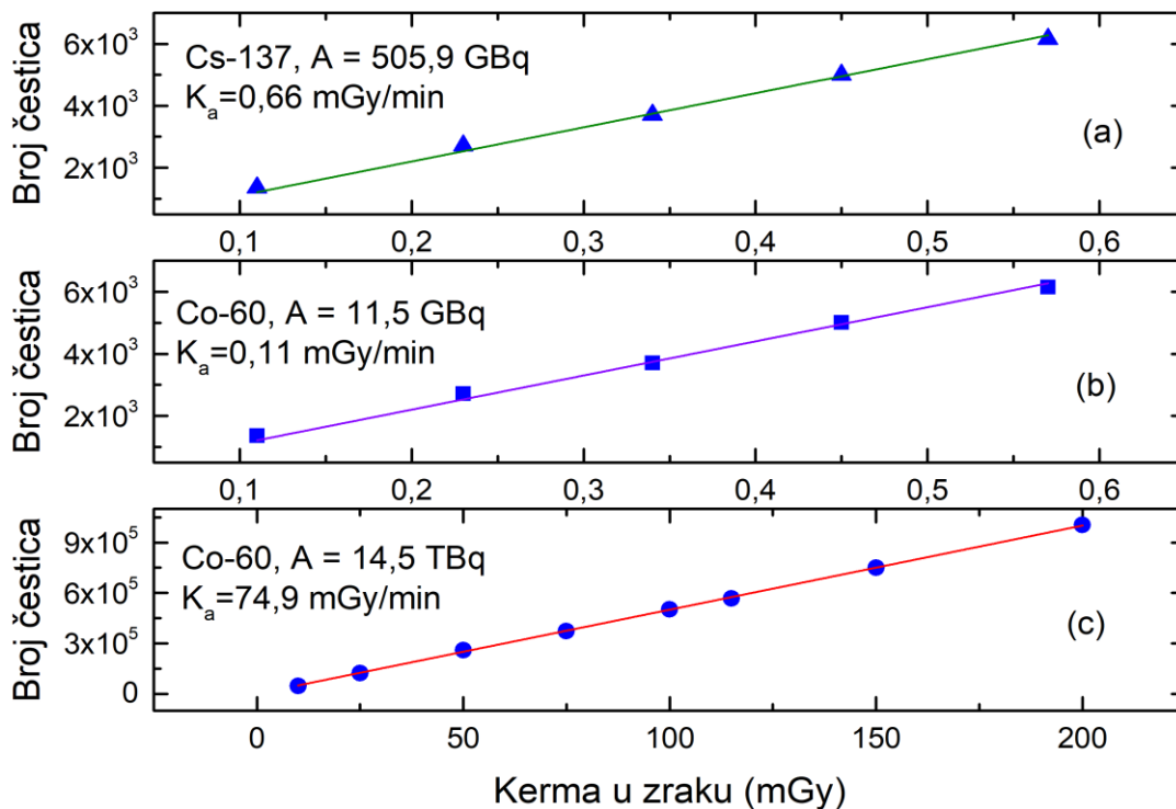
Slika 40. Odziv Schottkyjeve diode aktivne površine 2 \times 2 mm 2 na: (a) izvor 137 Cs aktivnosti 505,9 GBq, (b) izvor 60 Co aktivnosti 11,5 GBq i (c) izvor 60 Co aktivnosti 14,5 TBq.
