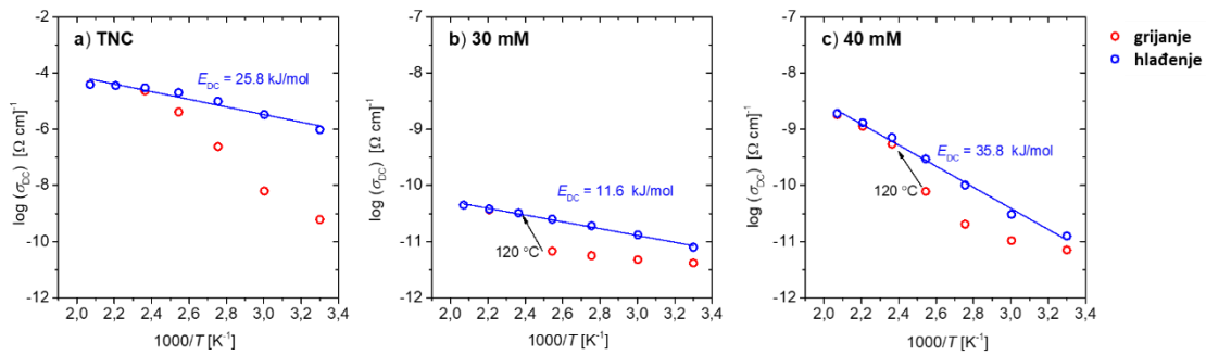
Slika 83. Prikaz temperaturne ovisnost DC vodljivosti ( \log(\sigma_{DC}) ) u režimima grijanja i hlađenja: a) nemodificiranih TNC i BTO/TNC kompozitnih uzoraka pripremljenih hidrotermalnom reakcijom b) 30 mM i c) 40 mM otopina \text{Ba}(\text{OH})_2 . Pravci su dobiveni modeliranjem eksperimentalnih podataka.
