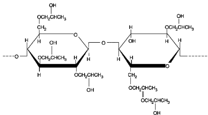
Slika 7. Struktura hidroksipropilceluloze 22
