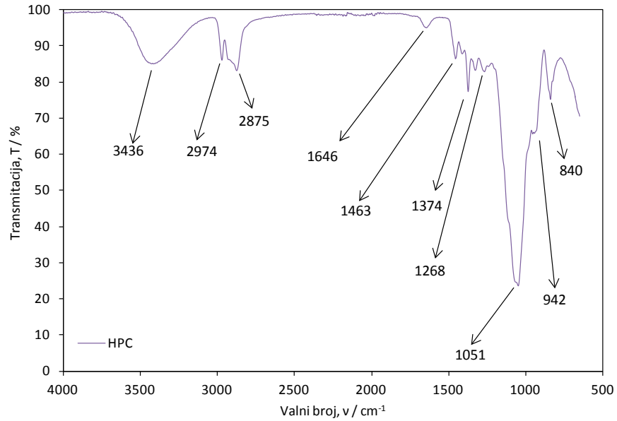
Slika 23. FTIR spektar HPC polimera
