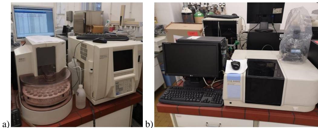
Slika 3.3. Uređaji korišteni TOC-V, Shimadzu a) i FTIR-ATR spektrometar b)
