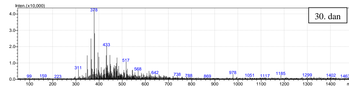
Slika 4.4. Rezultati LC/MS analize biorazgradnje polistirena za 3.,7.,14.,21. i 30. dan za pokus T15.
