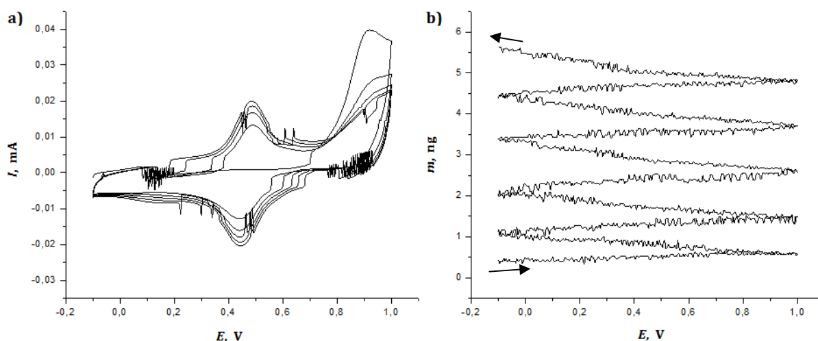
Slika 4.1. a) Ciklički voltamogram i b) pripadajuća promjena mase kroz 5 ciklusa u prvom ispitivanju 1. elektrode u 1 M H 2 SO 4 , pri brzini promjene potencijala od 50 mV/s.
