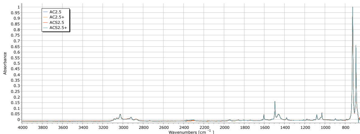
Slika 71. Snimljeni FTIR spektar za uzorak dobiven reakcijom n=5 u reaktorima ispisanima od PrimaCreator UV/VIS Clear smole.
