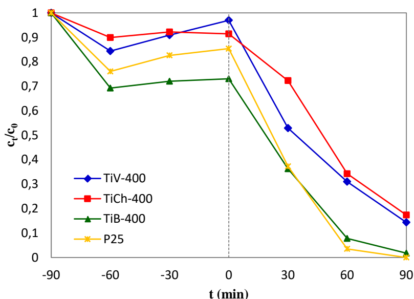
Slika 4.20. Koncentracija AB25 bojila nakon adsorpcije i tijekom fotokatalitičke razgradnje s TiB 400, TiCh 400, TiV 400 katalizatorima pri UVA zračenju ( \gamma_{RR45}=30 mg/l, \gamma_{kat}=1 g/l, pH =6,8).
