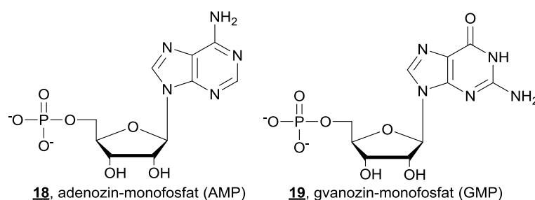
Slika 16. Strukture purinskih nukleotida AMP i GMP
