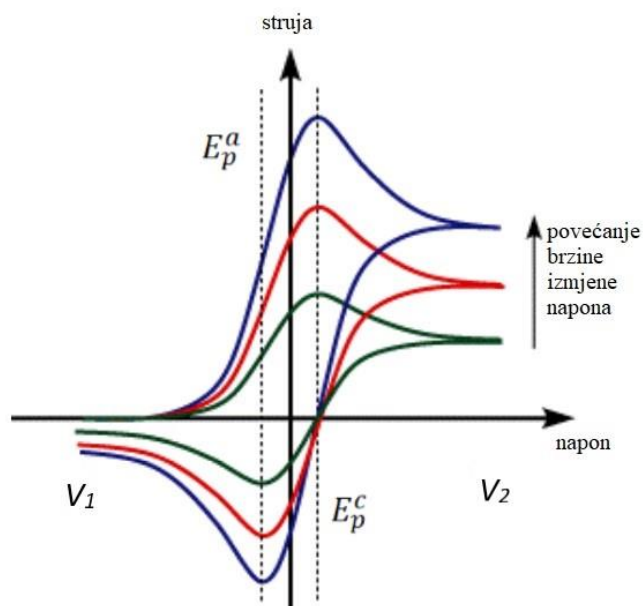
Slika 2.5. Tipičan izgled voltamograma za jednoelektronsku reverzibilnu reakciju [19]
