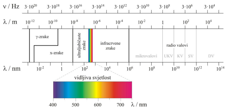
Slika 6. Elektromagnetski spektar.
