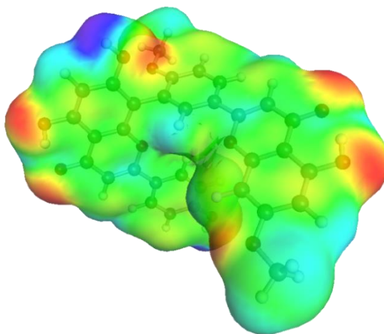
Slika 7. Energetski i geometrijski optimirana molekula ginkgetina
