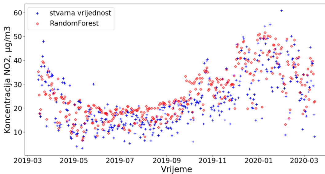
Slika 5.6. Prikaz stvarnih vrijednosti u usporedbi sa Random Forest modelom grupirane kao srednje vrijednosti po danu
