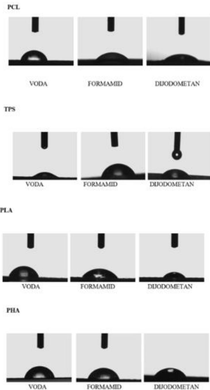
Slika 40. Kapljice testnih kapljevine na čistim polimernim materijalima PCL, PLA, TPS i PHA
