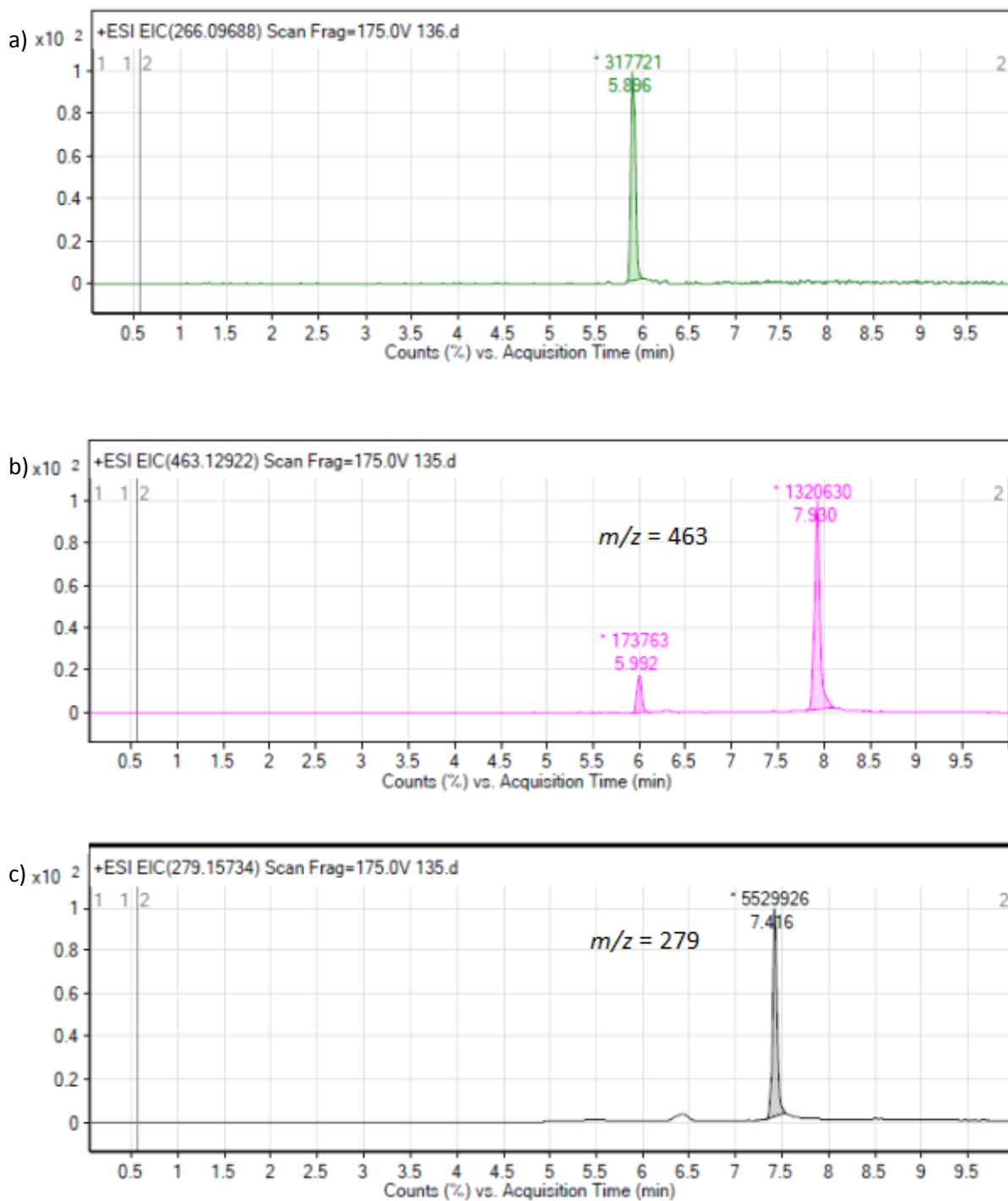
Slika 29. Kromatogram ALB prije hidrolize (a), nastali razgradni produkt m/z 463 (b), te razgradni produkt m/z 279 nakon 24 h eksperimenta
