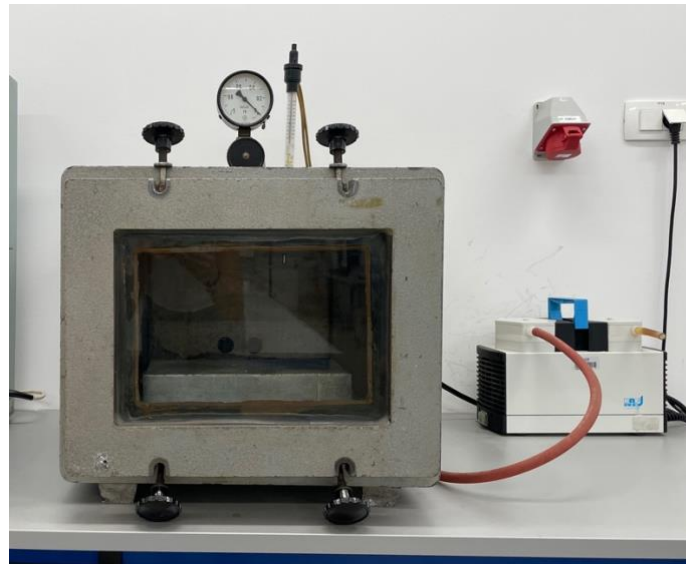
Slika 14. Vakuum sušionik
